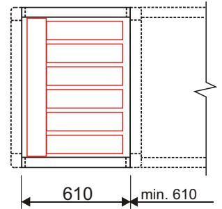
AKF Aktivkohle- filterteil
